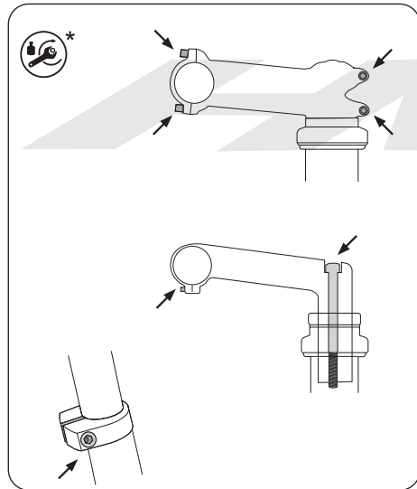
Mögliche Positionen von Schraubverbindungen zur Anpassung
