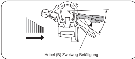
Hebel (B) Zweiweg-Betätigung
