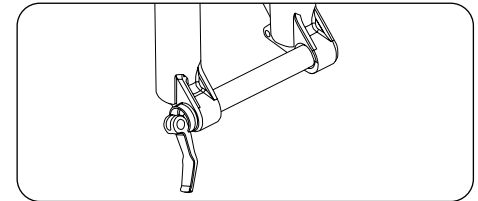
Steckachse in den Gabelausfallenden, ohne Nabe, Rock Shox® Gabel
