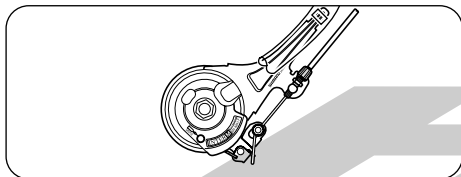
Rollenbremse
